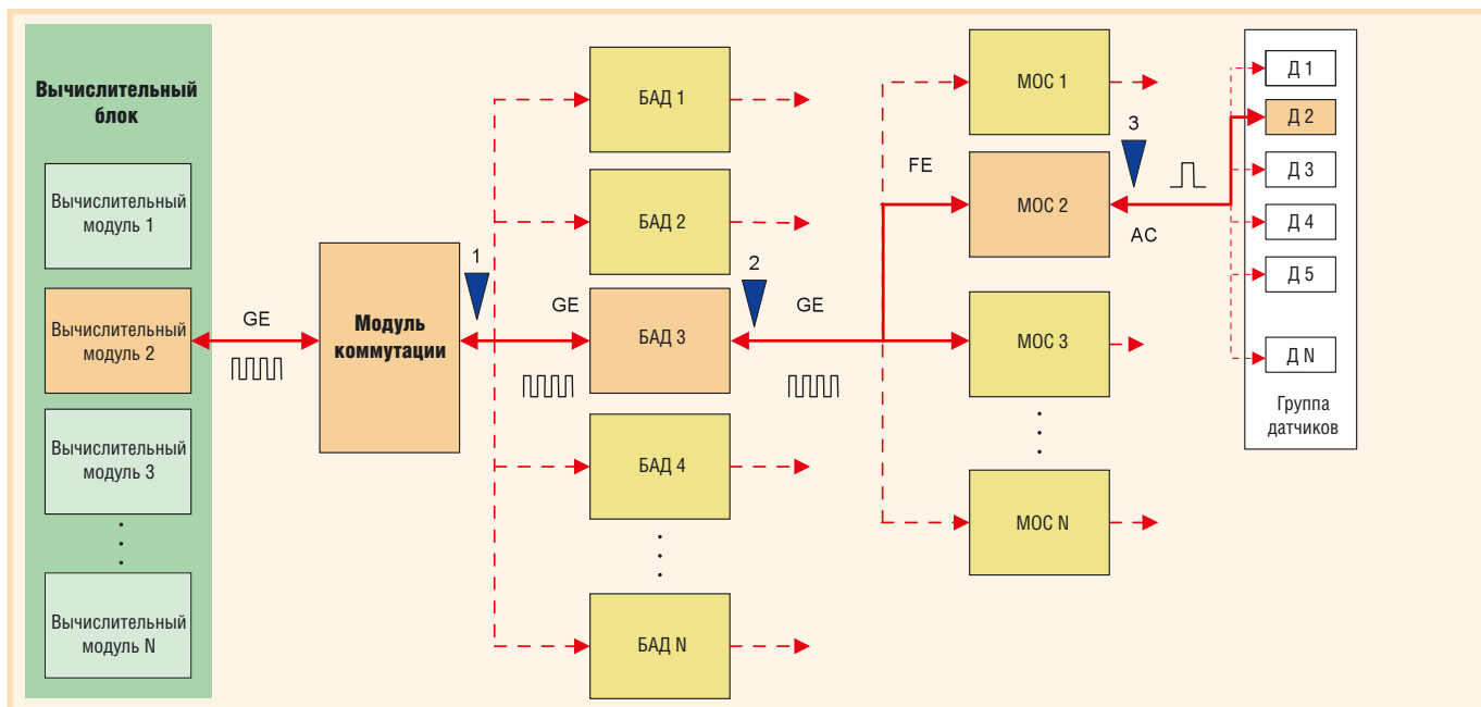
Условные обозначения: — синхропоследовательность; — импульс дискретизации; FE — канал Fast Ethernet; GE — канал Gigabit Ethernet; n — номер способа синхронизации внешних устройств в перечне; AC — аналоговый сигнал; Д — датчик; МОС — модуль обработки сигналов; БАД — блок агрегирования данных.
