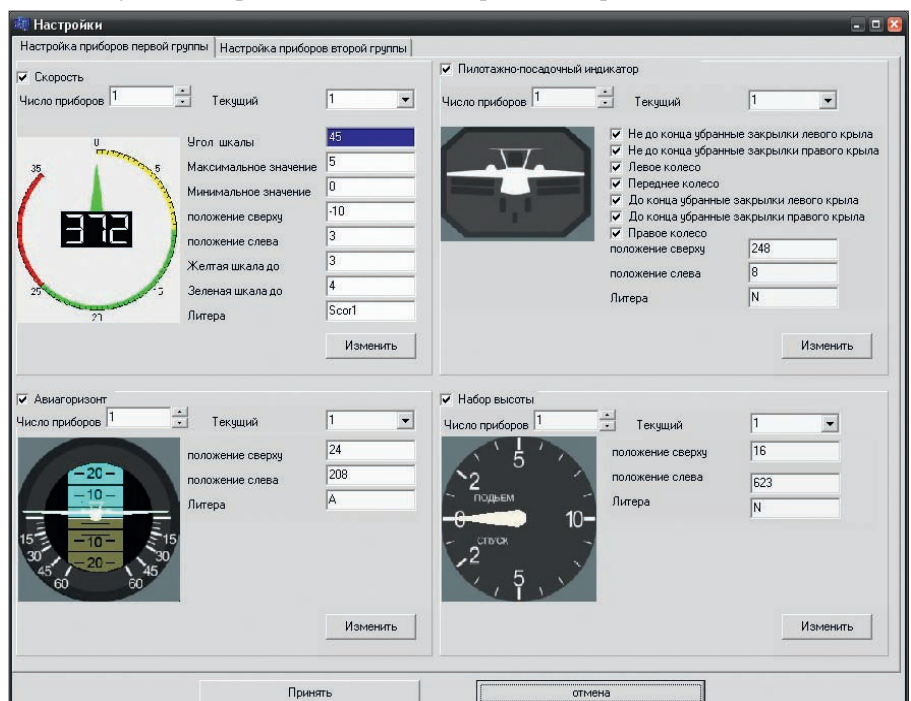
Рис. 9. Внешний вид экрана настроек программы ВДП
