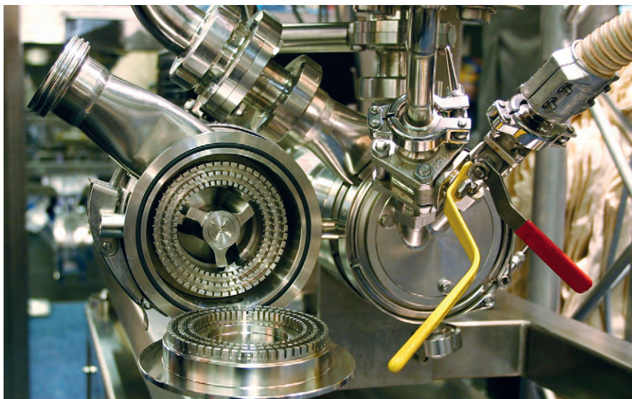
Рис. 1. Система диспергирования с TDS (компания Ystral)
