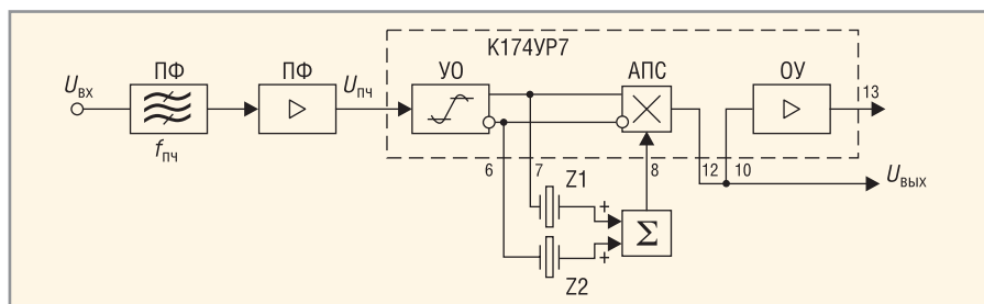
Рис. 1. Структурная схема тракта демодулятора сигналов F1B с малой девиацией частоты
