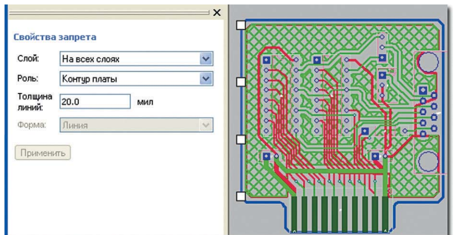
Рис. 18. Создание контура печатной платы
