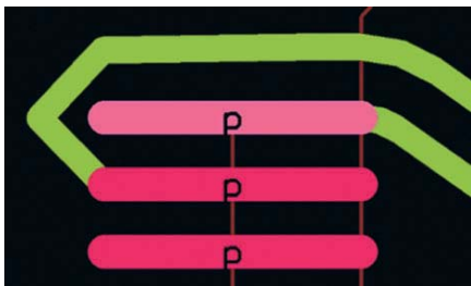
Рис. 10. Выделение функционально эквивалентных контактов
