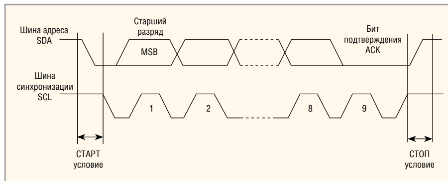
Рис. 2. Временная диаграмма одной посылки интерфейса I 2 C
